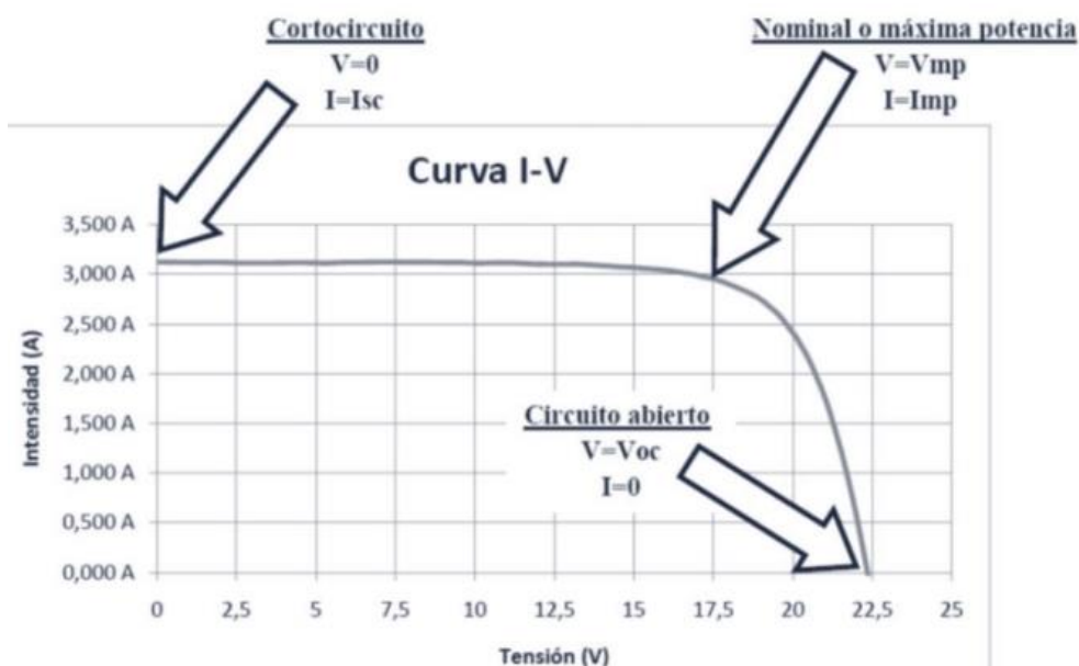
Fig. 7 Curva I-V captador solar [3]
