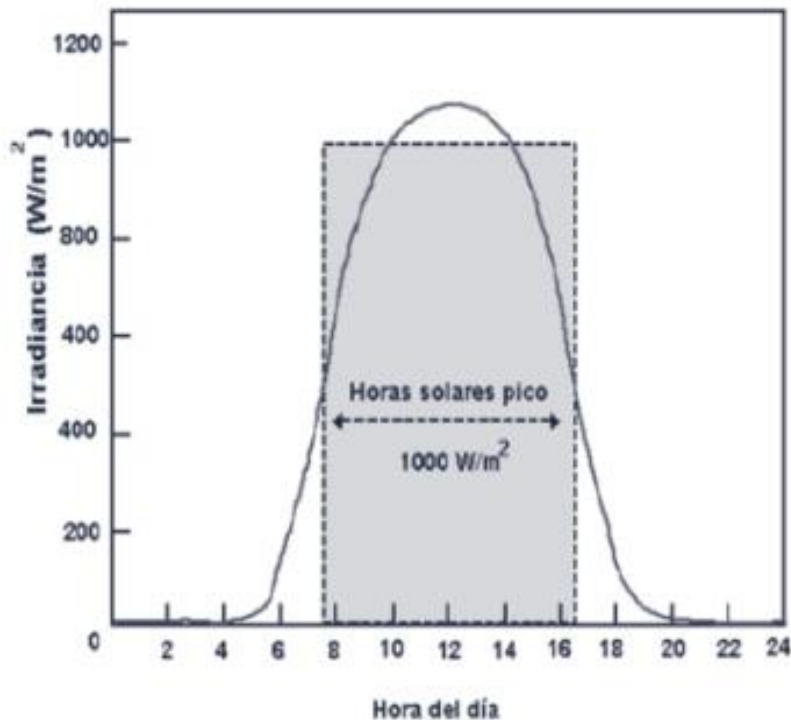
Fig. 6 Hora solar pico [3]
