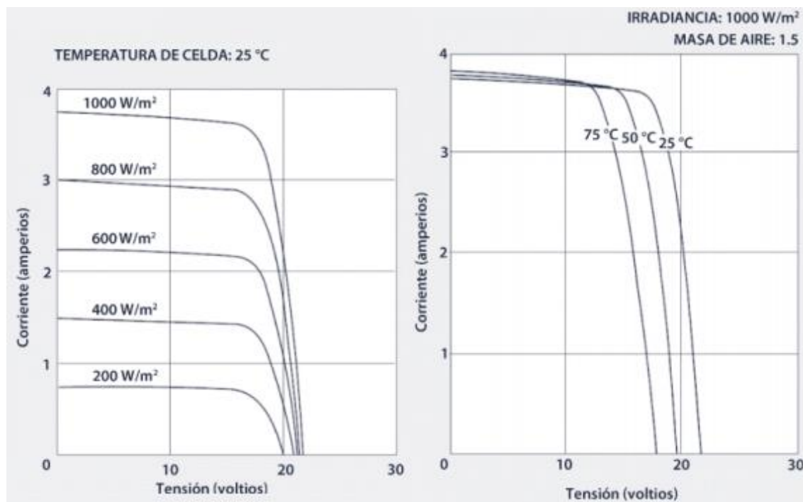
Fig. 8 Curvas I-V dependientes de la irradiación y temperatura [3]
