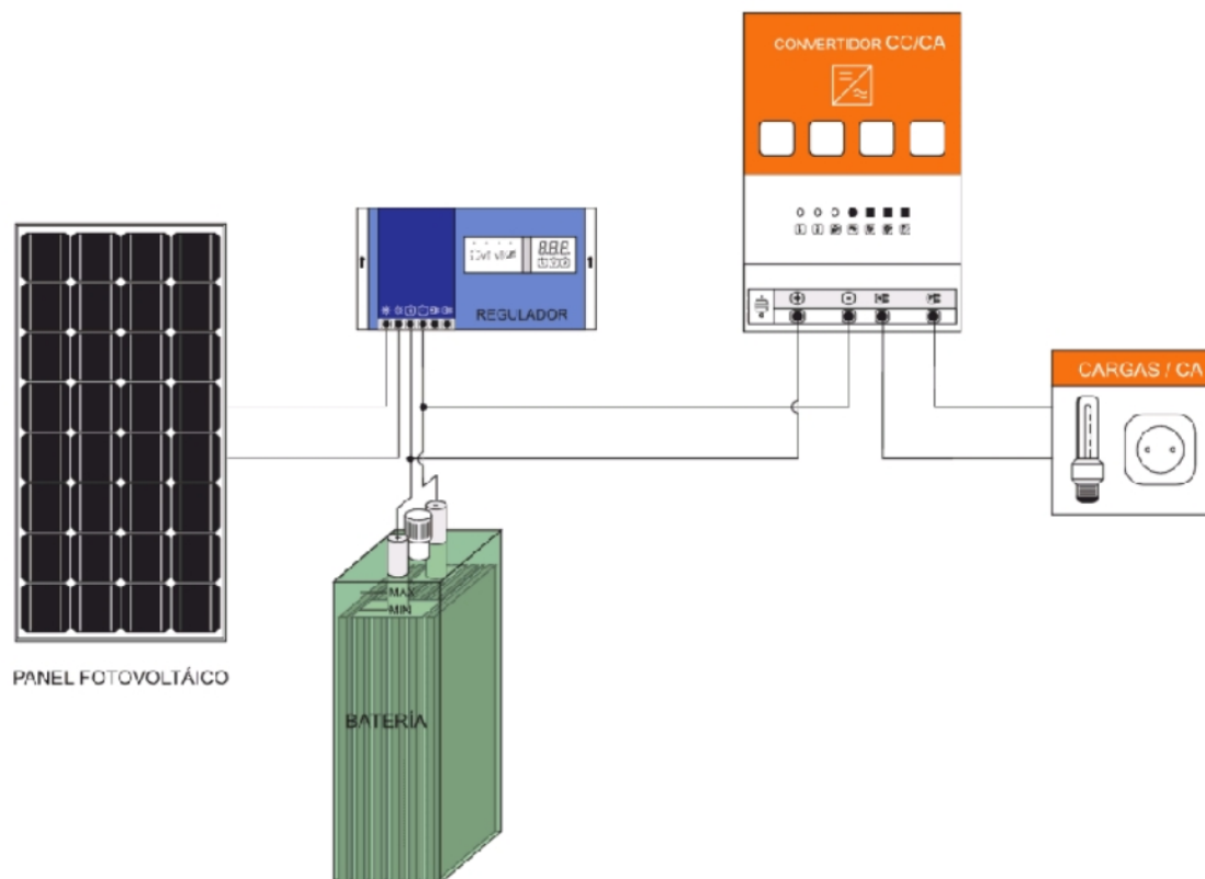
Fig. 10 Configuración típica para sistemas fotovoltaicos aislados con acumulación [26]
